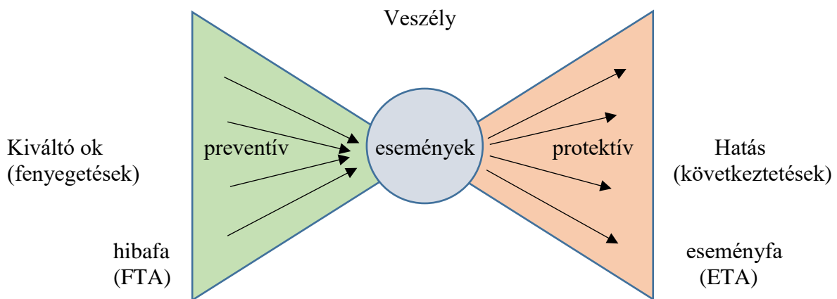
24. ábra, Bow-tie modell alapján (saját szerkesztés)
